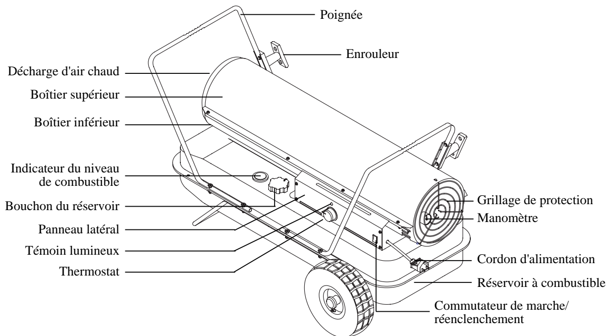
Illustration 2. Modèle DFA-170C / 210C
