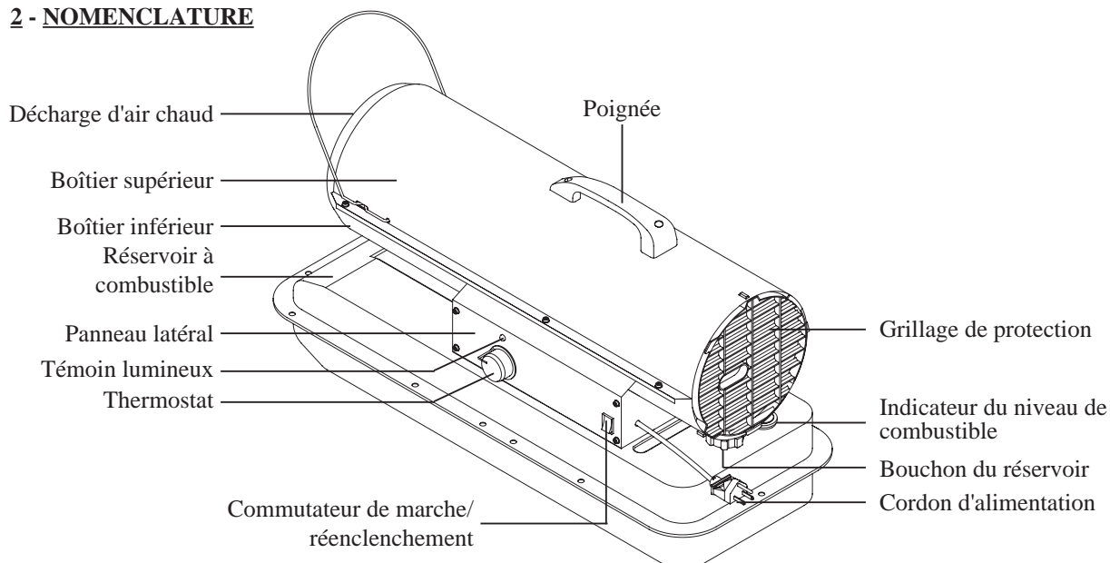
Illustration 1. Modèle DFA-45T / DFA-70T
