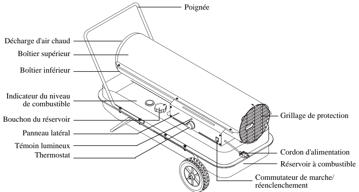
Illustration 2. Modèle DFA-125T
