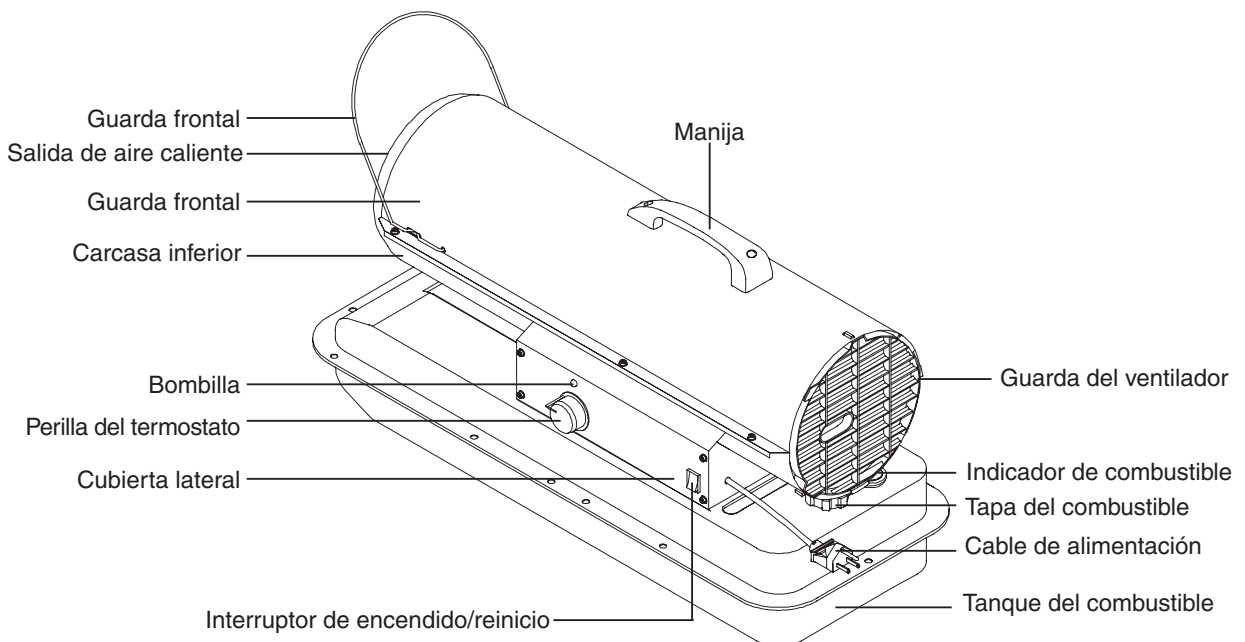
Figura 1. MODELOS DFA-45T / DFA-70T
