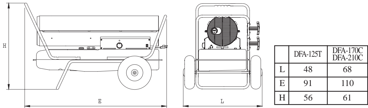
DFA-125T / DFA-170C / DFA-210C
