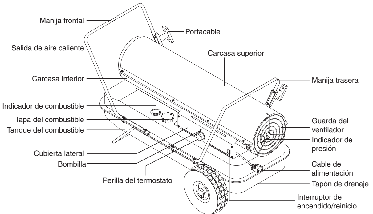
Figura 3. MODELOS DFA-170C/210C
