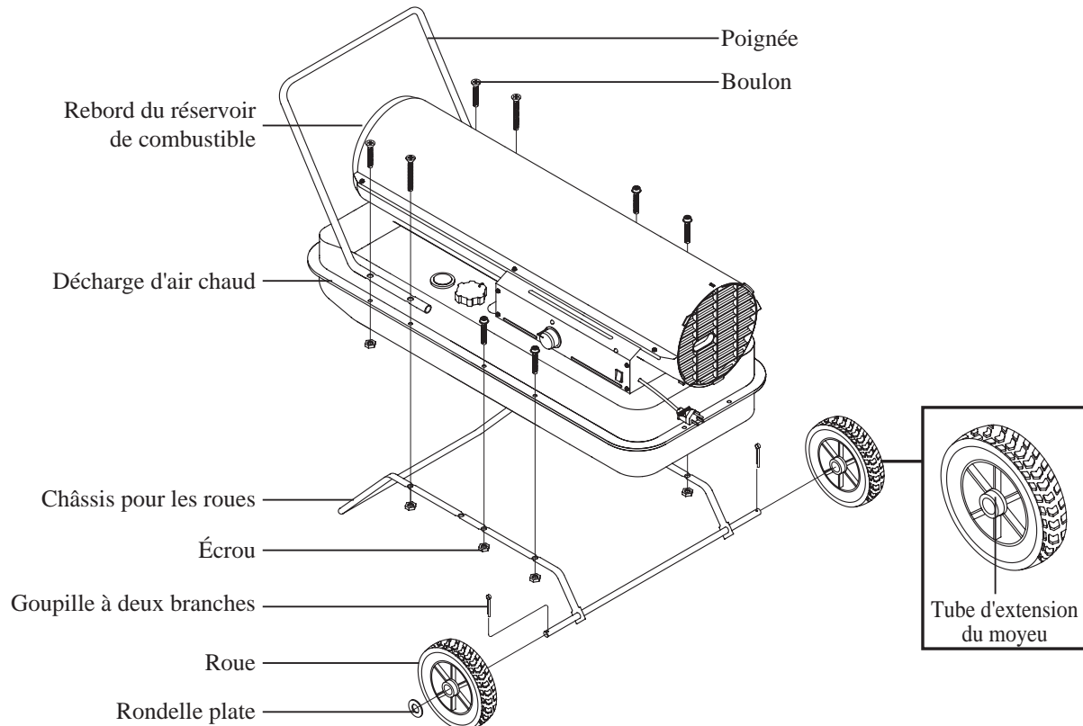
Illustration 6. Montage des roues et de la poignée pour les modèles DFA-125T seulement.
