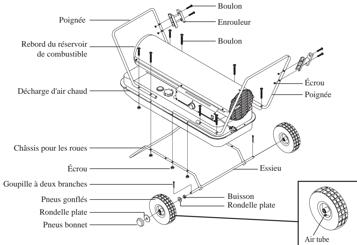
Illustration 7. Montage des roues et de la poignée pour les èles DFA-170C/210C seulement.
