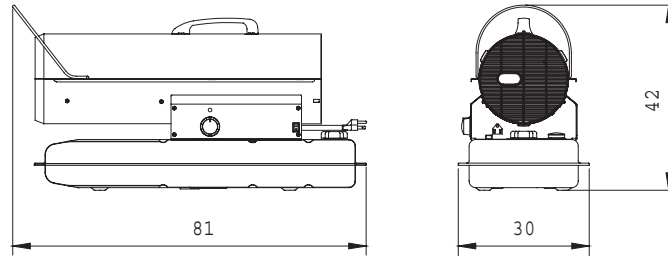
DFA-45T / DFA-70T
