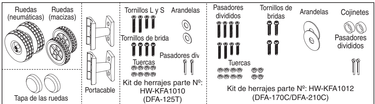
Figura 5. Modelos DFA-125T / DFA-170C / DFA-210C
