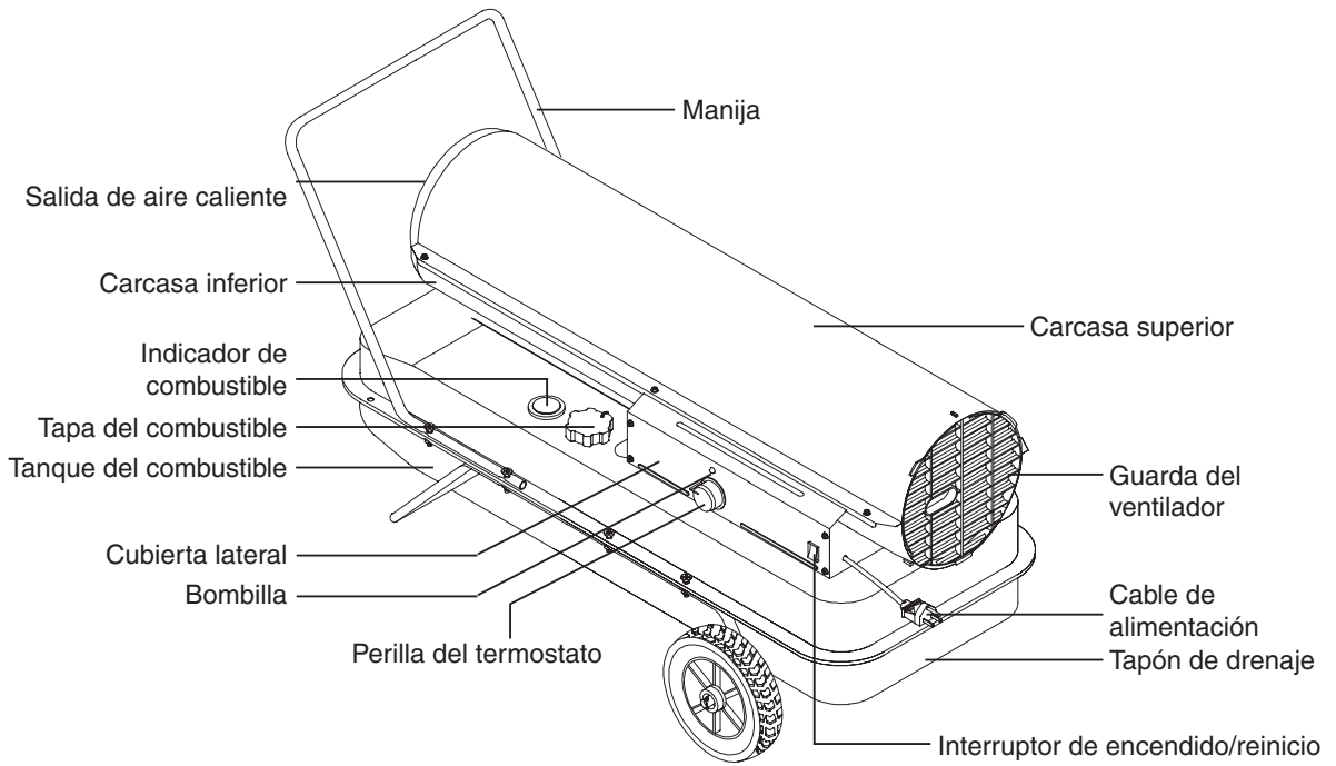
Figura 2. MODELO DFA-125T
